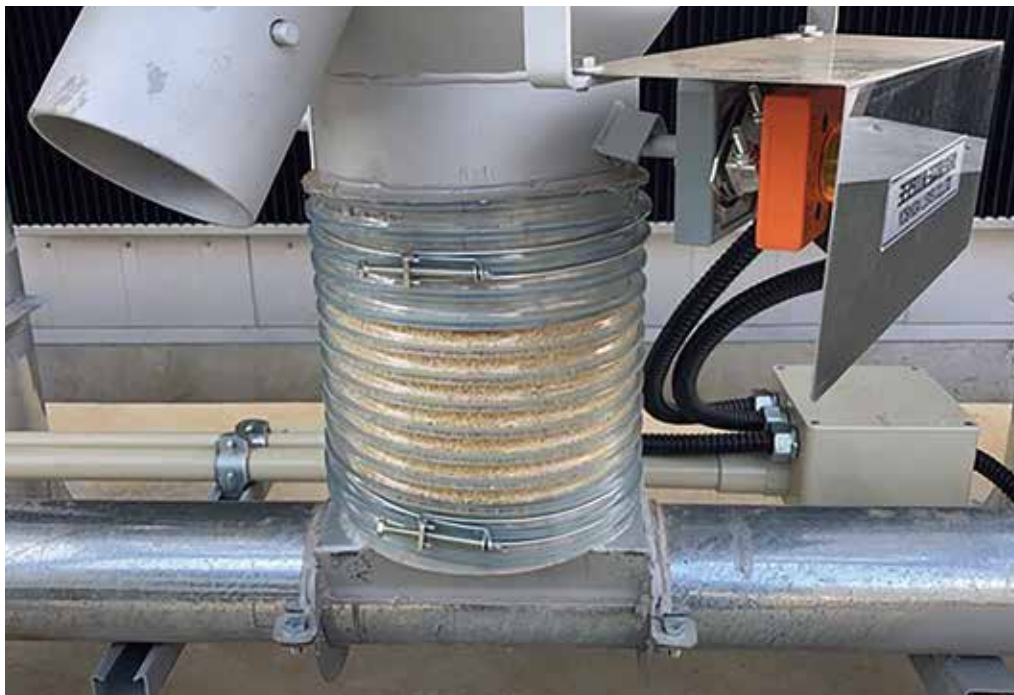
タンク自動切り換え装置
